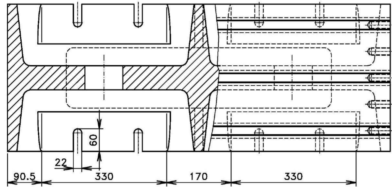
ČÁST.ŘEZ A-A
